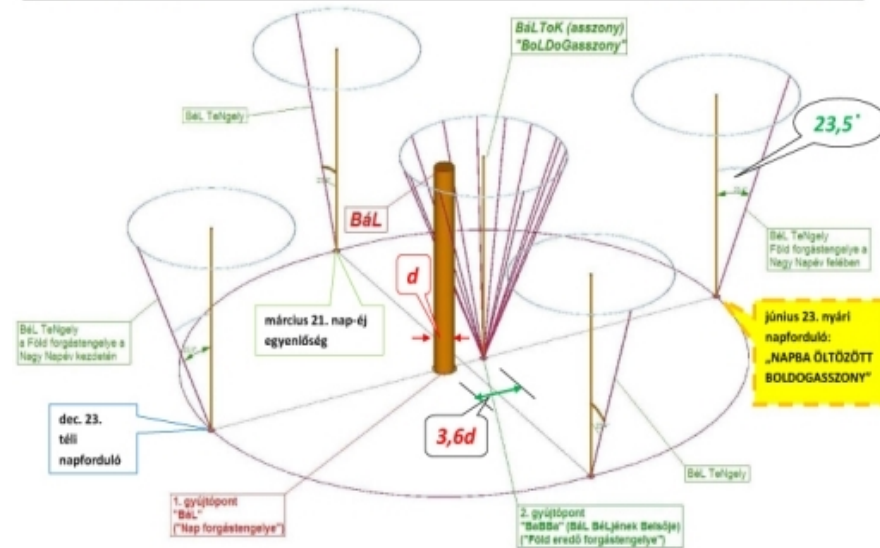
A precessziós kúp a Nagy Napév 25920 éve alatt zárul. A kúp alkotója a Föld forgástengelye .
